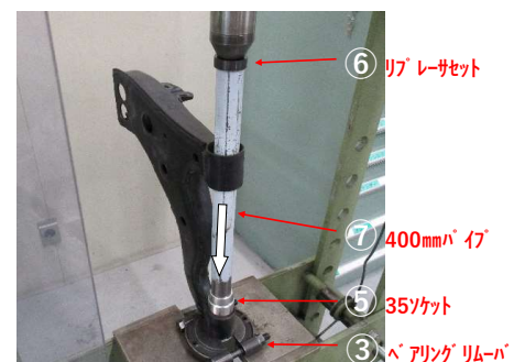
6. No.2ブシはパイプ⑦を使って抜く。
