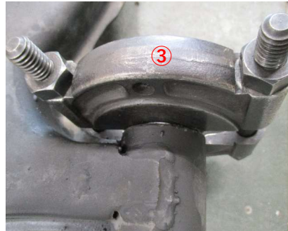
2. 起こしたブシのフランジとアームの間にベアリングリムバ③を取り付ける。
