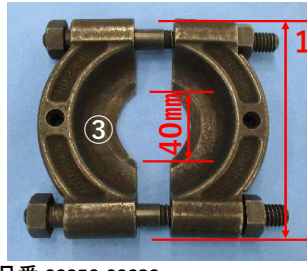
品番:09950-00020 ベアリングリムバ
