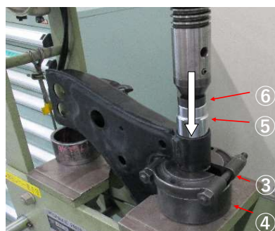
5. No.1ブシを抜く。
